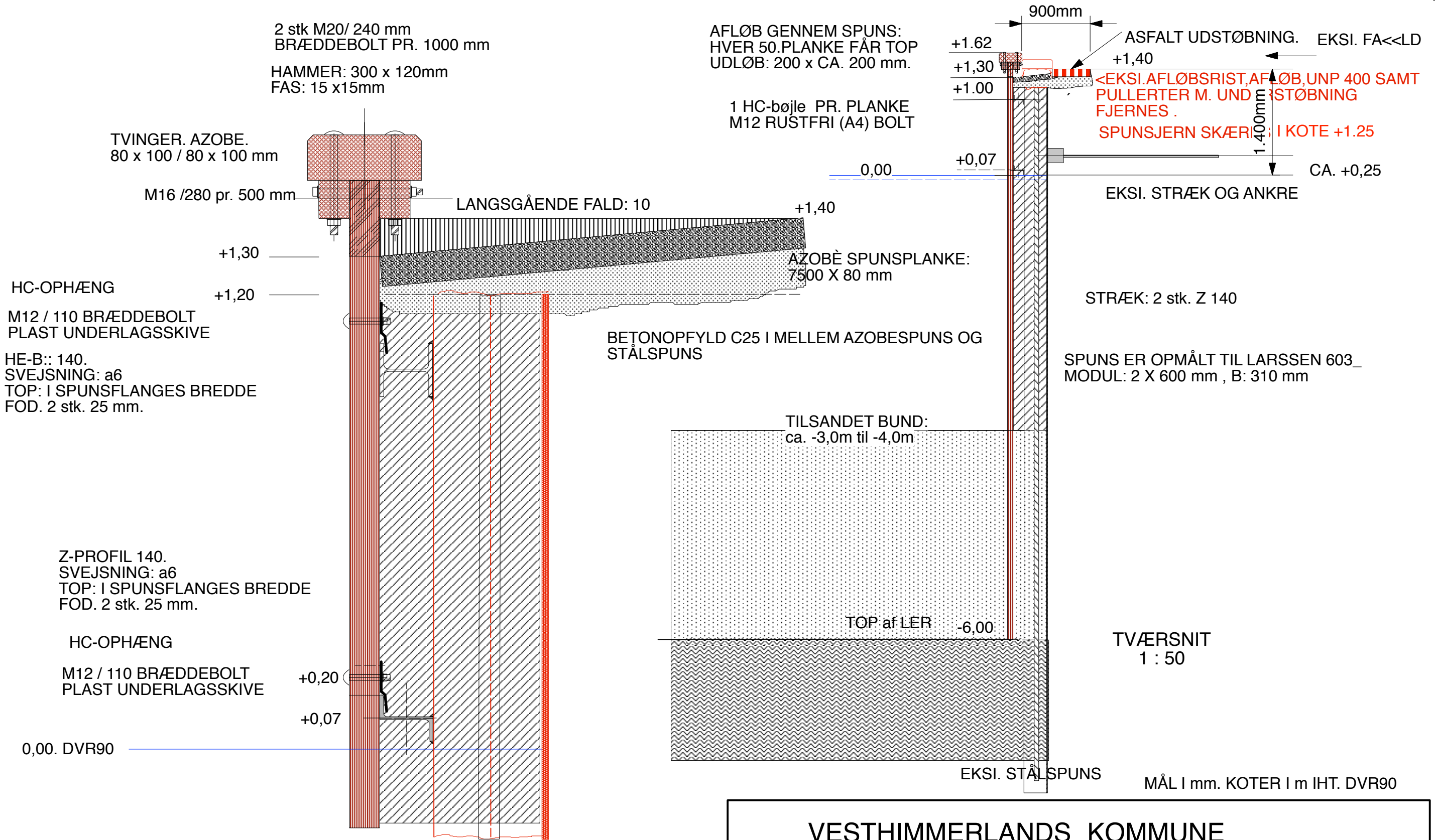
DETALJE AF AFVANDING OG OPHÆNG 1 : 10
